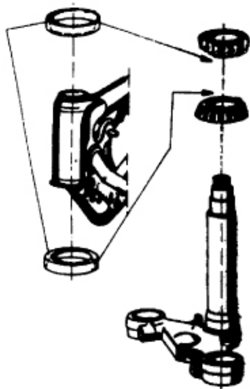
Umrüstset auf Kegelrollenlager
